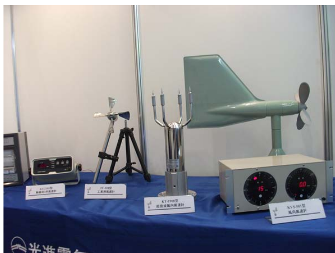
超音波式風向風速計、工業用風速計他
